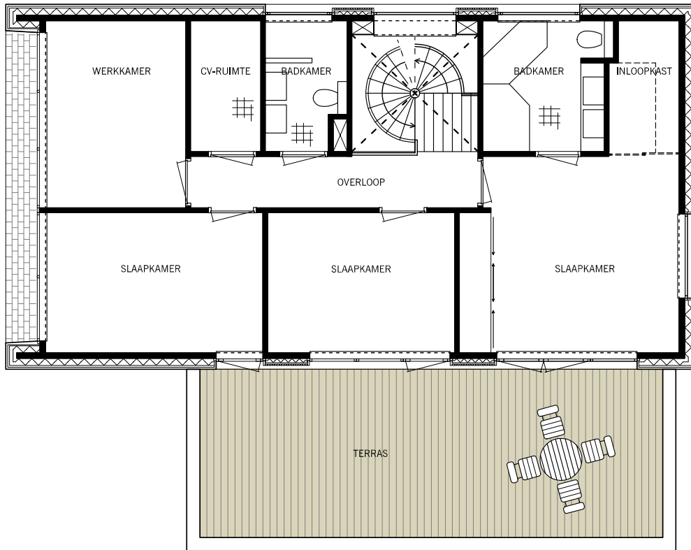
Eerste verdieping
