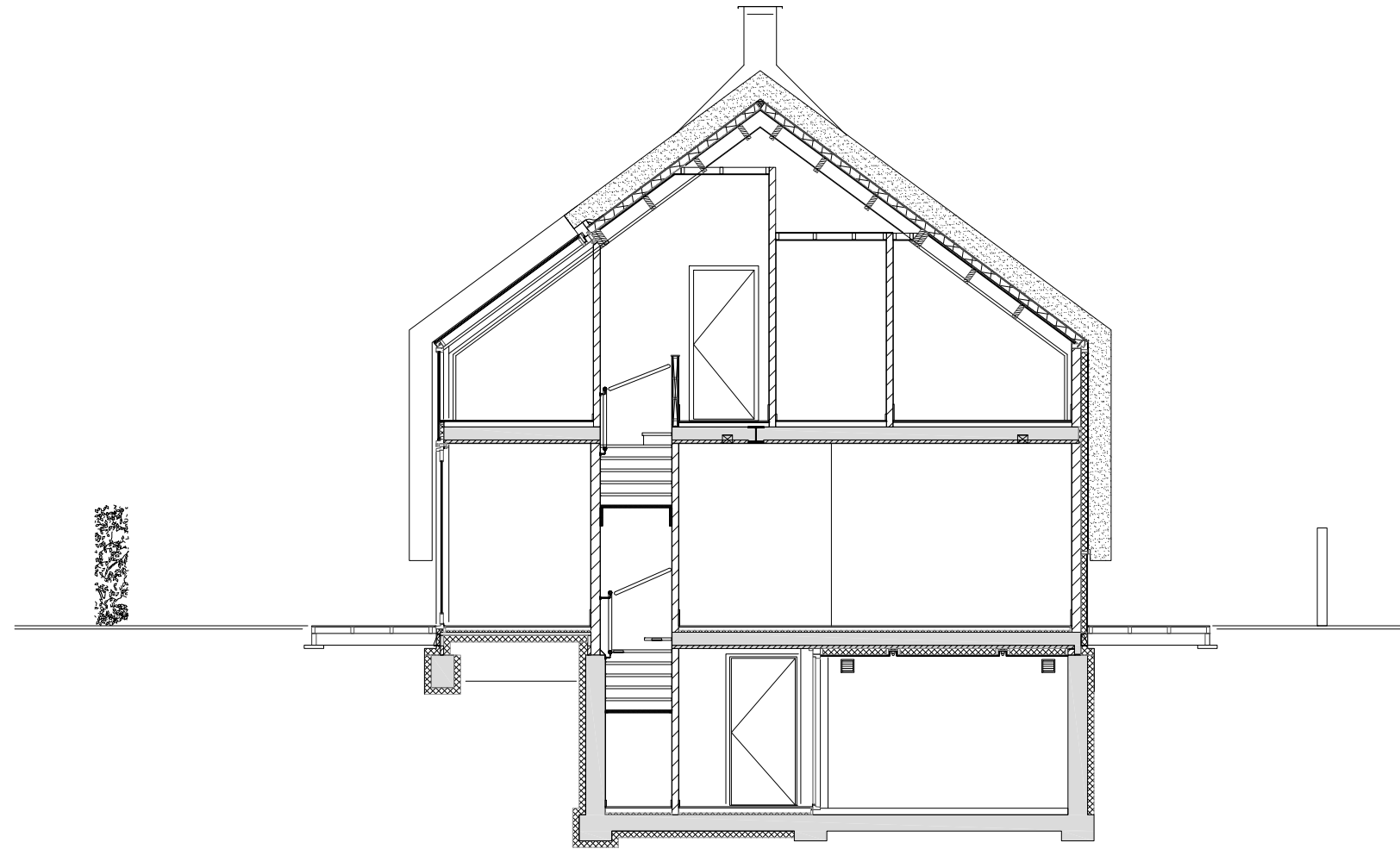
Section 01
