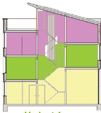
Variant 1 3 laags, dakterras straatzijde
