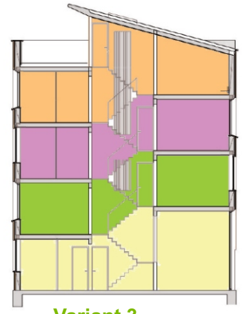
Variant 3 4 laags, dakterras straatzijde
