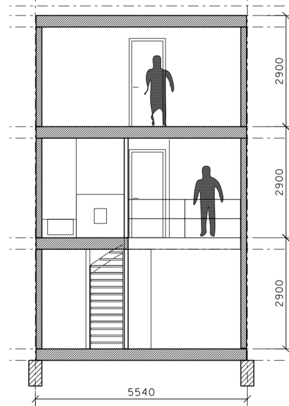
dwarsdoorsnede
