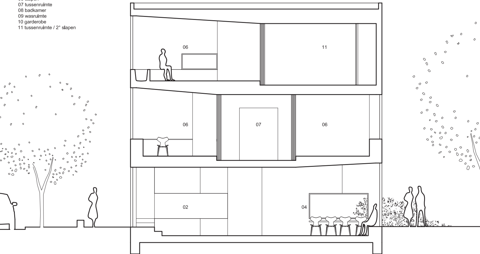
DOORSNEDE A VRIJSTAAND HUIS
