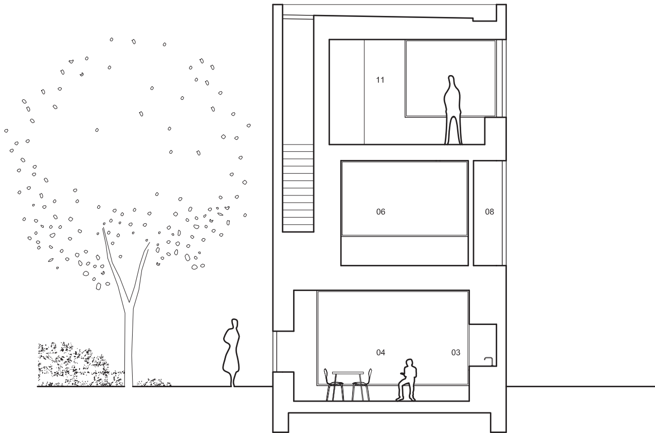
DOORSNEDE B VRIJSTAAND HUIS
