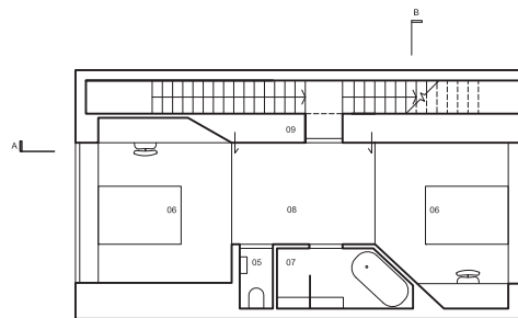
1E VERDIEPING
