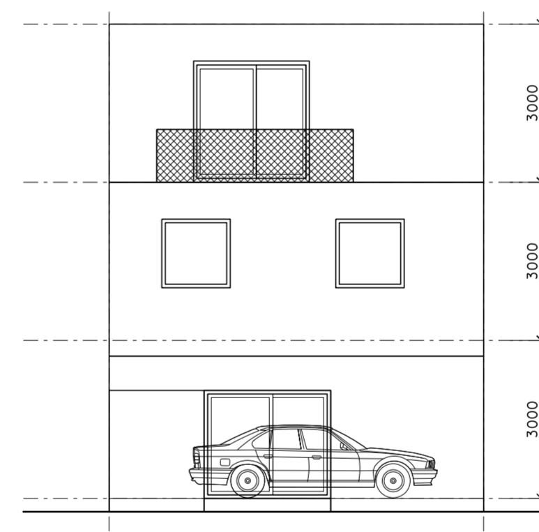
linker zijgevel
