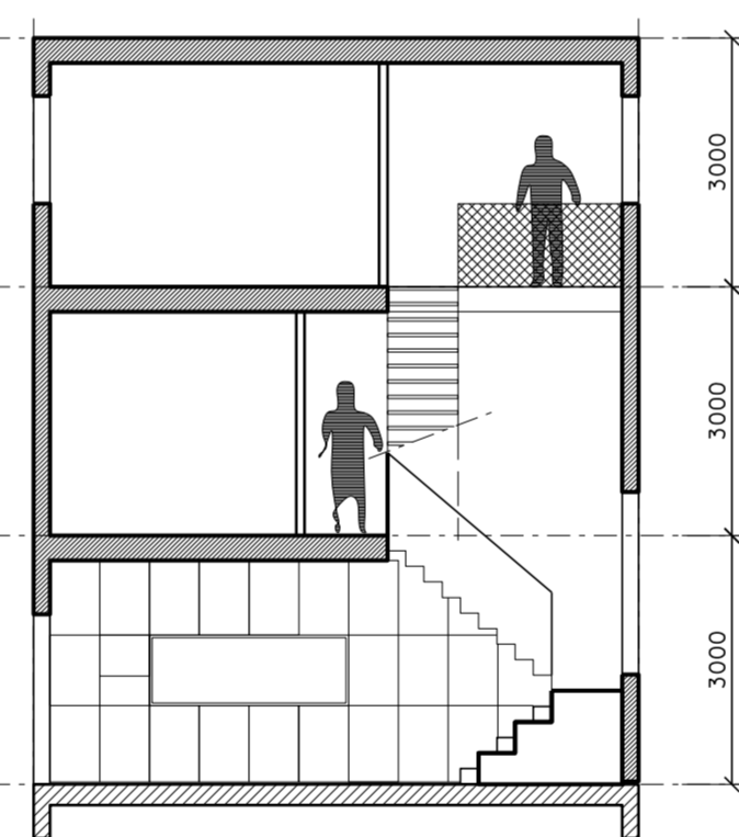
doorsnede BB
