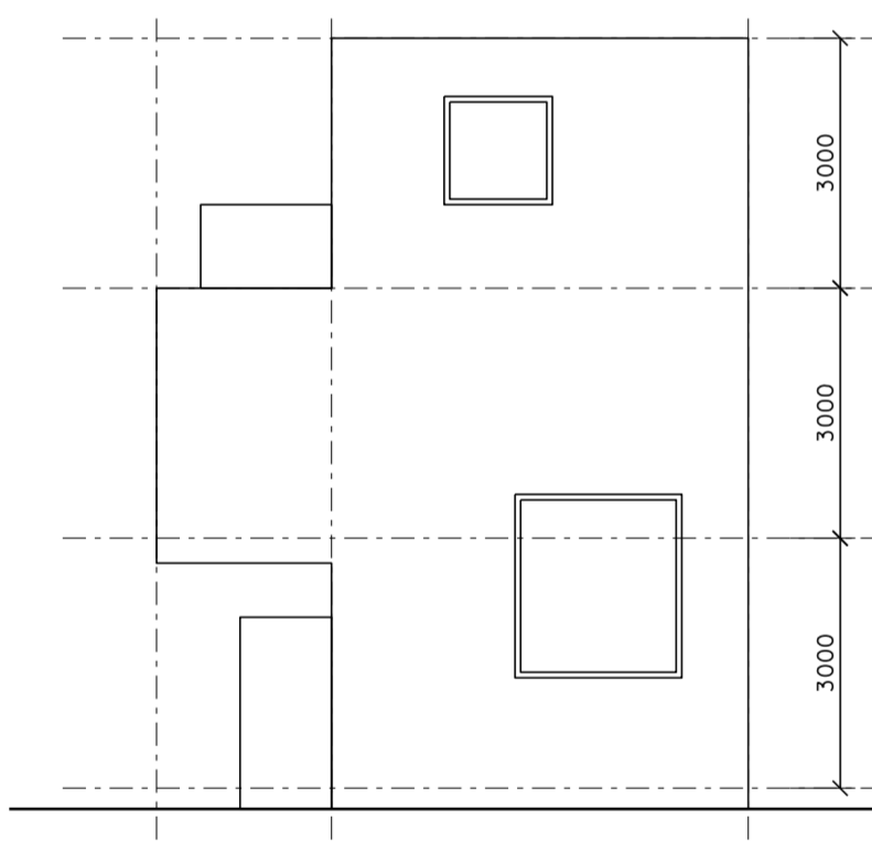
voorgevel
