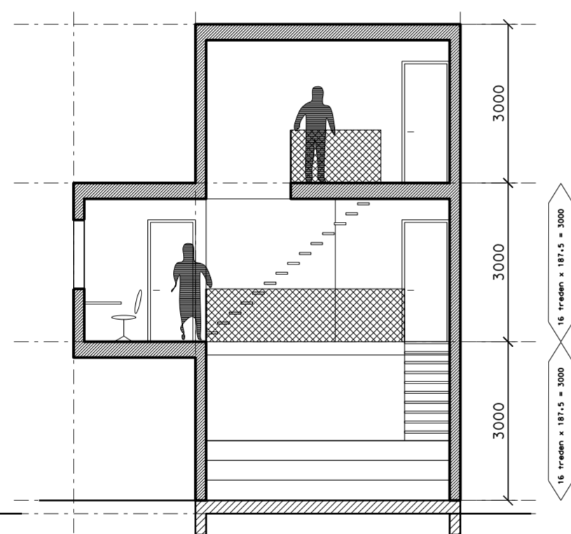
doorsnede AA
