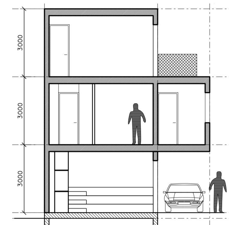
doorsnede CC
