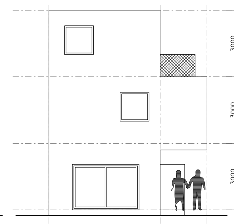
achtergevel
