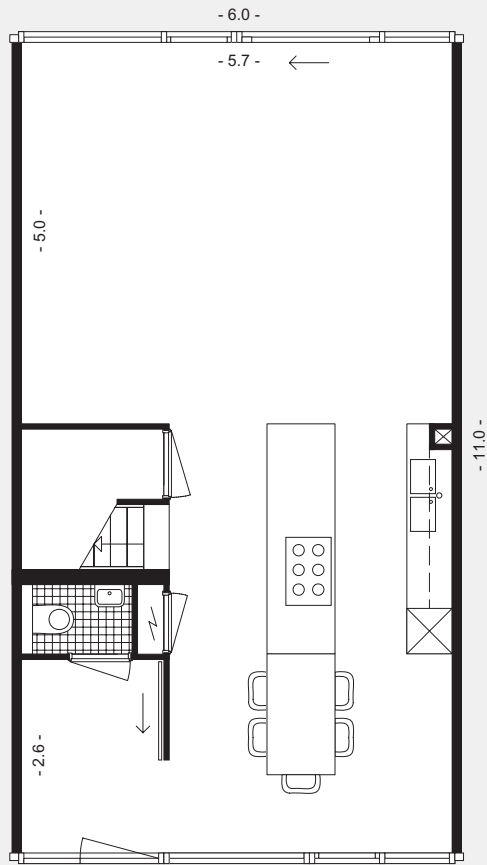
Begane grond 1:100
