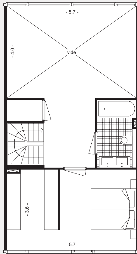
Eerste verdieping
