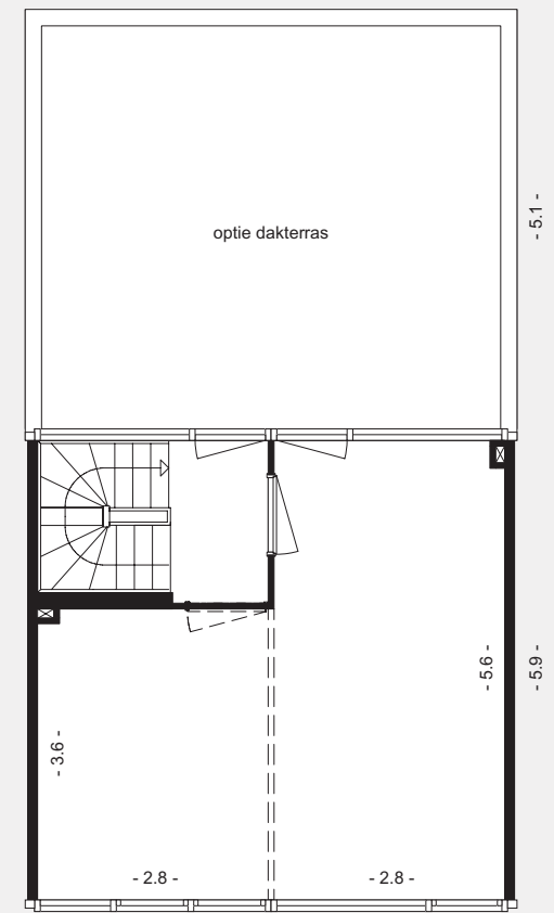
Tweede verdieping
