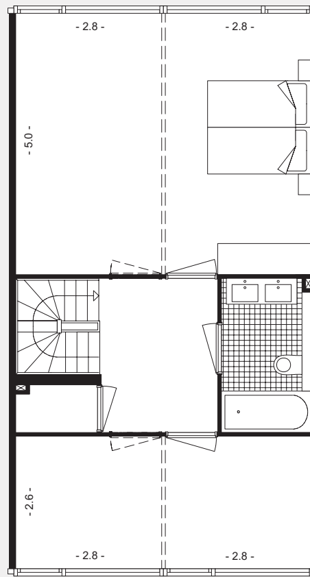
Eerste verdieping
