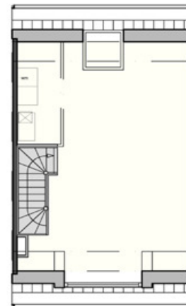
dakopbouw 2, volledige zolder 2E VERDIEPING
