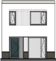
Voorgevel IJBURGHUIS 1
