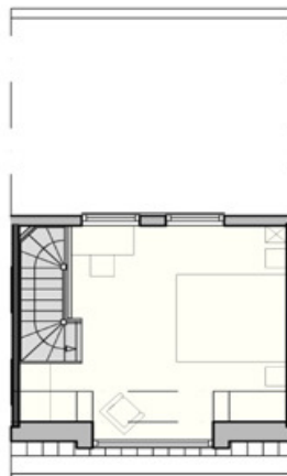
dakopbouw 1, over de 1/2 verdiepings-diepte 2E VERDIEPING
